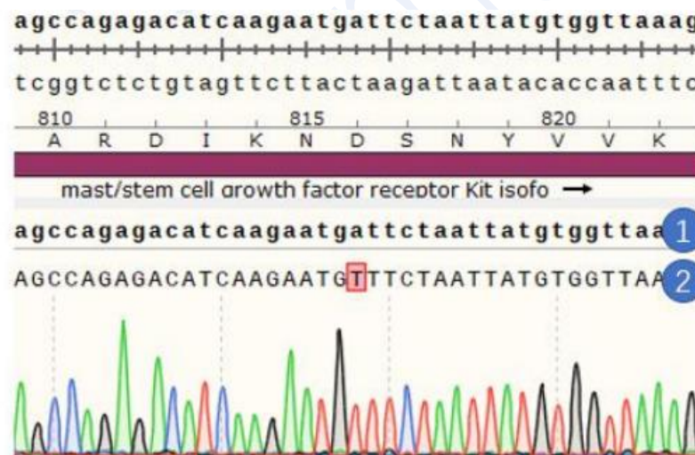
Fig . Sanger 测序验证结果
